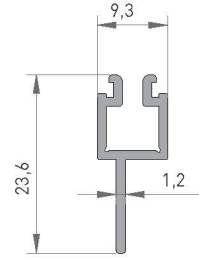
5408 DERZ ÇITA 0.155 kg/mt
