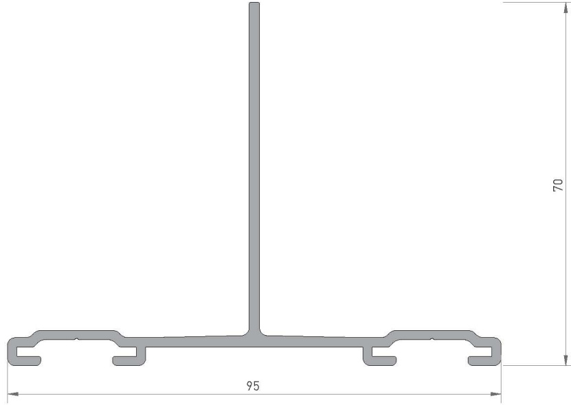
3818 TAŞIYICI "T" PRF. 0.995 kg/mt
