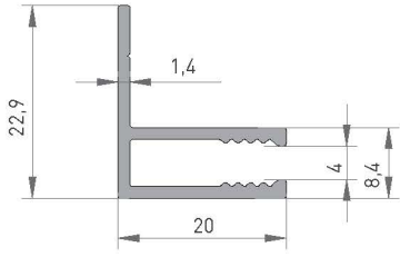
4706 KOMPOZİT " F " PROFİL 0.240 kg/mt
